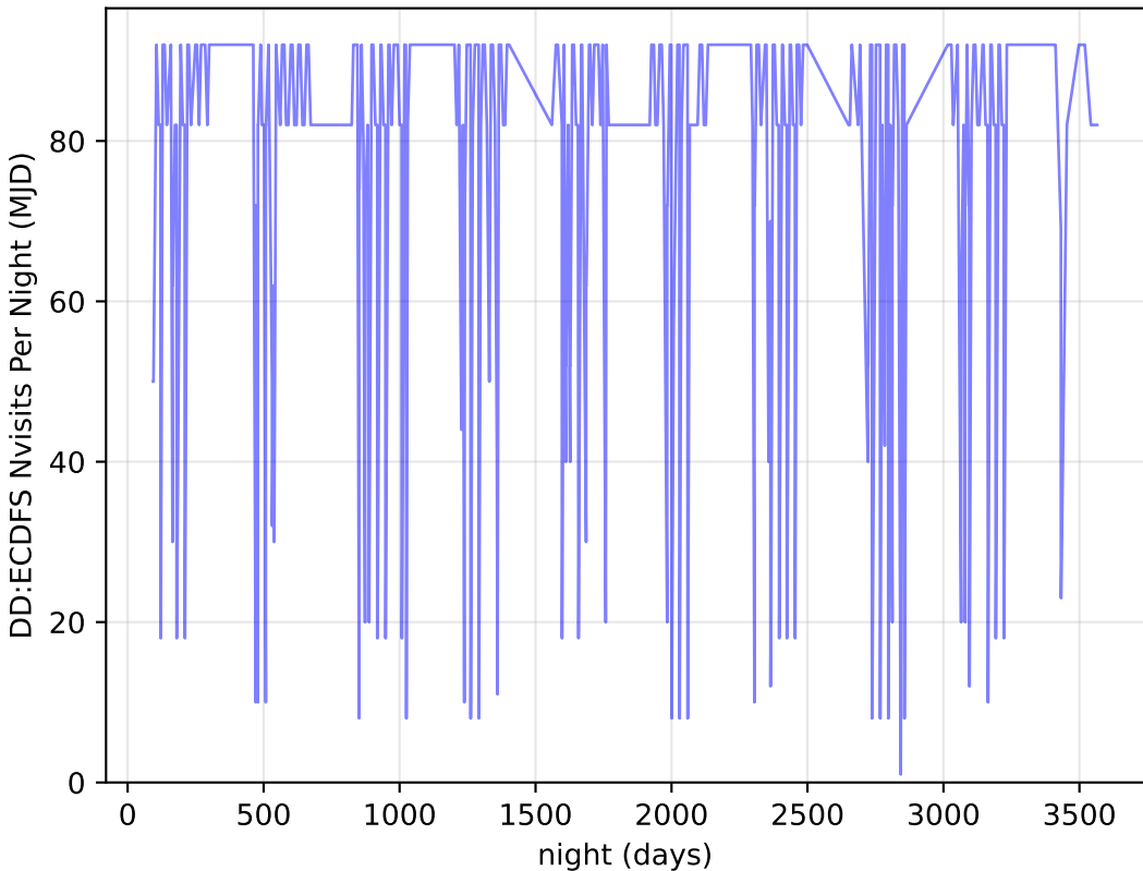
extra_ss_neo2_v3.4_10yrs all bands: DD:ECDFS Nvisits Per Night
