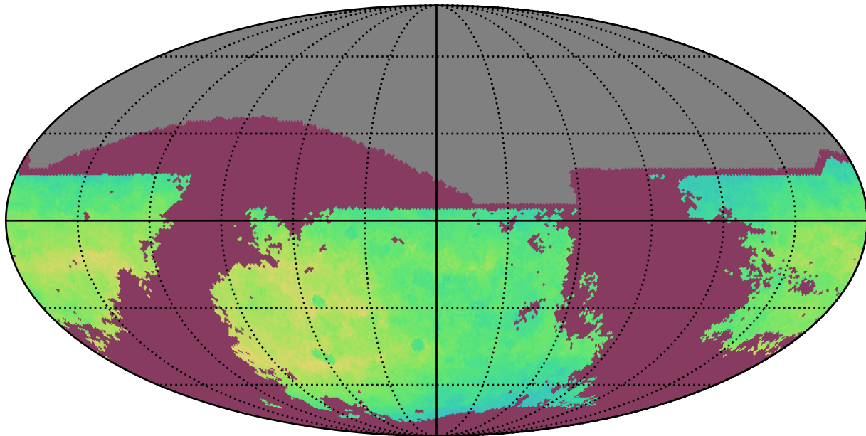
early_u_fpextra4.0_v3.4_10yrs i: NgalScale
