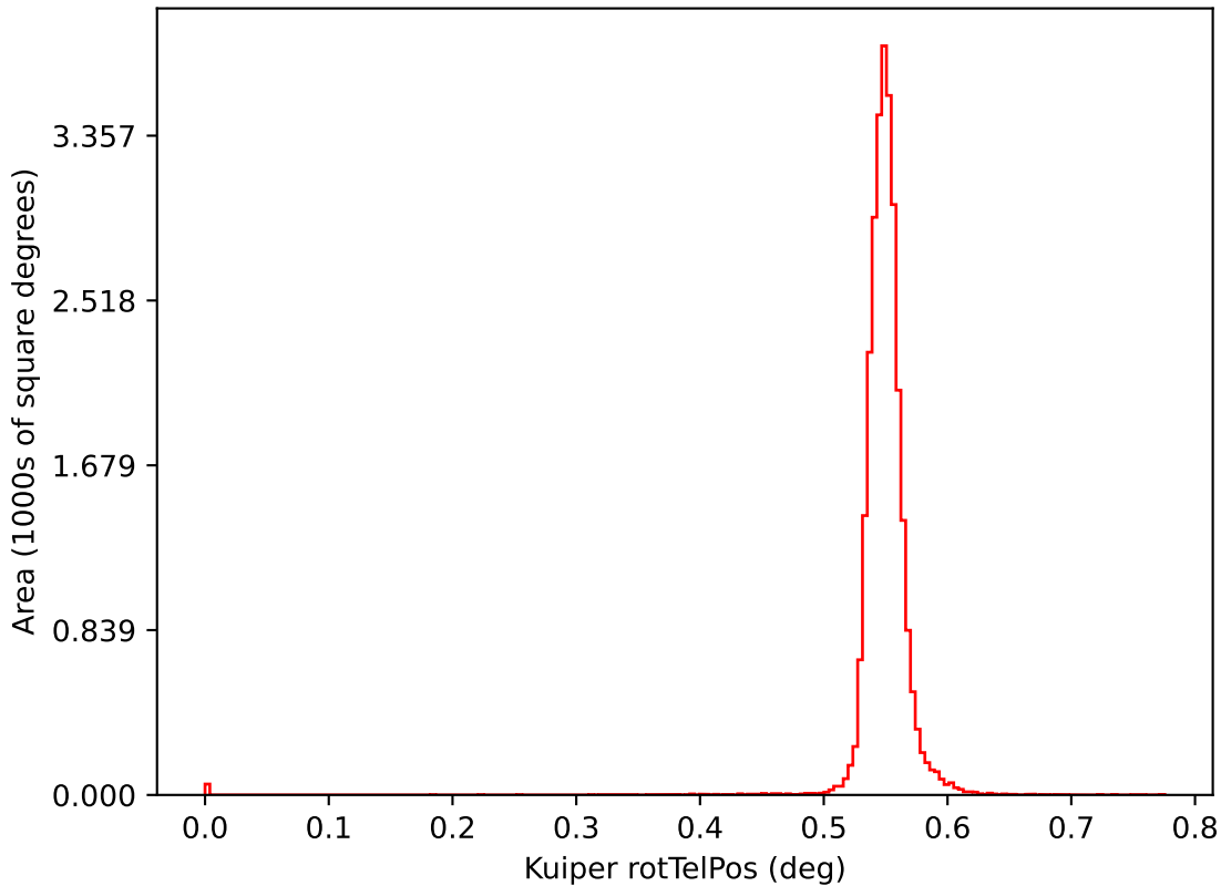
early_u_fpextra4.0_v3.4_10yrs i: Kuiper rotTelPos
