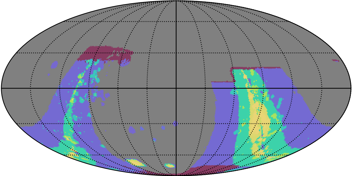
early_u_fpextra4.0_v3.4_10yrs : GalplaneFootprintMetric_combined_map_Tau_46_5
