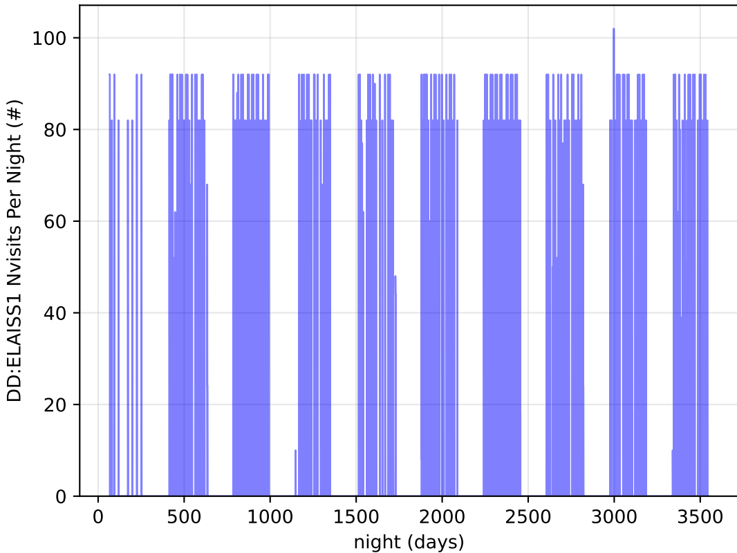
early_u_fpextra4.0_v3.4_10yrs all bands: DD:ELAISS1 Nvisits Per Night
