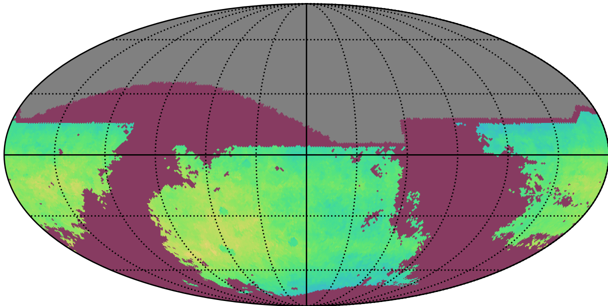
early_u_fpextra3.0_v3.4_10yrs i: NgalScale
