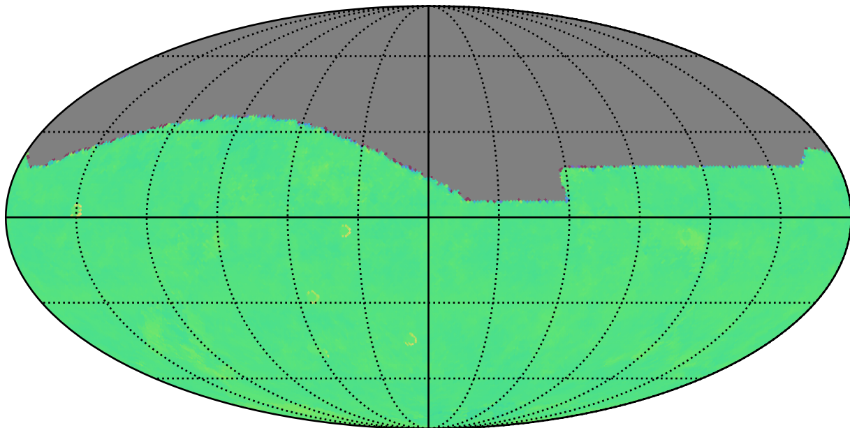
early_u_fpextra3.0_v3.4_10yrs i: Kuiper rotTelPos
