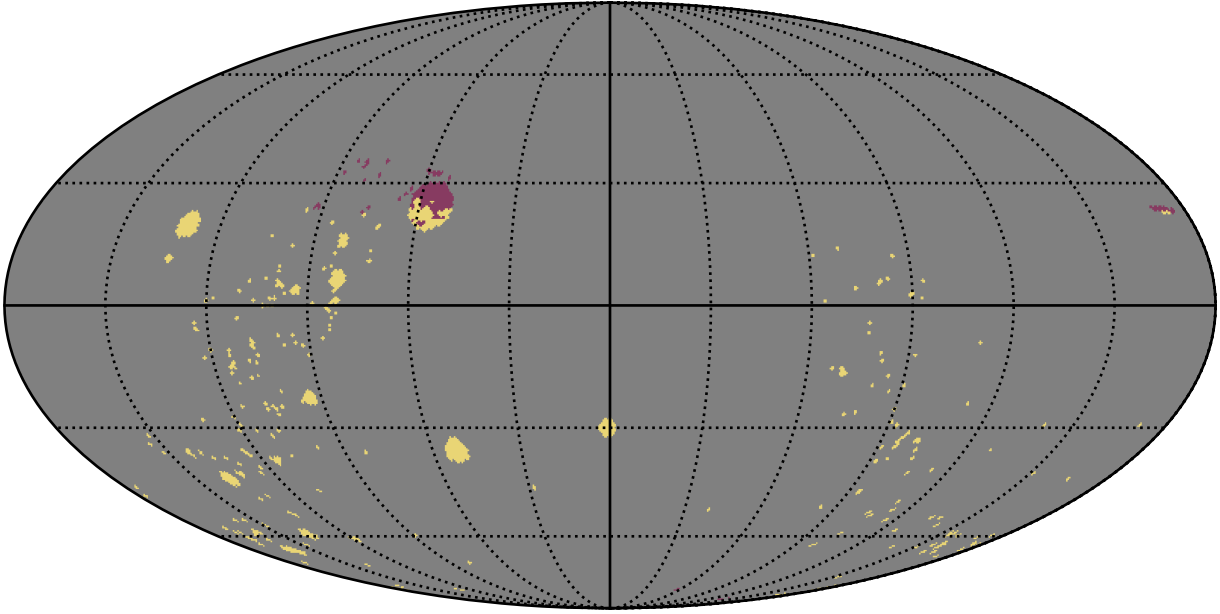
early_u_fpextra3.0_v3.4_10yrs : GalplaneFootprintMetric_open_clusters_map_Tau_46_5
