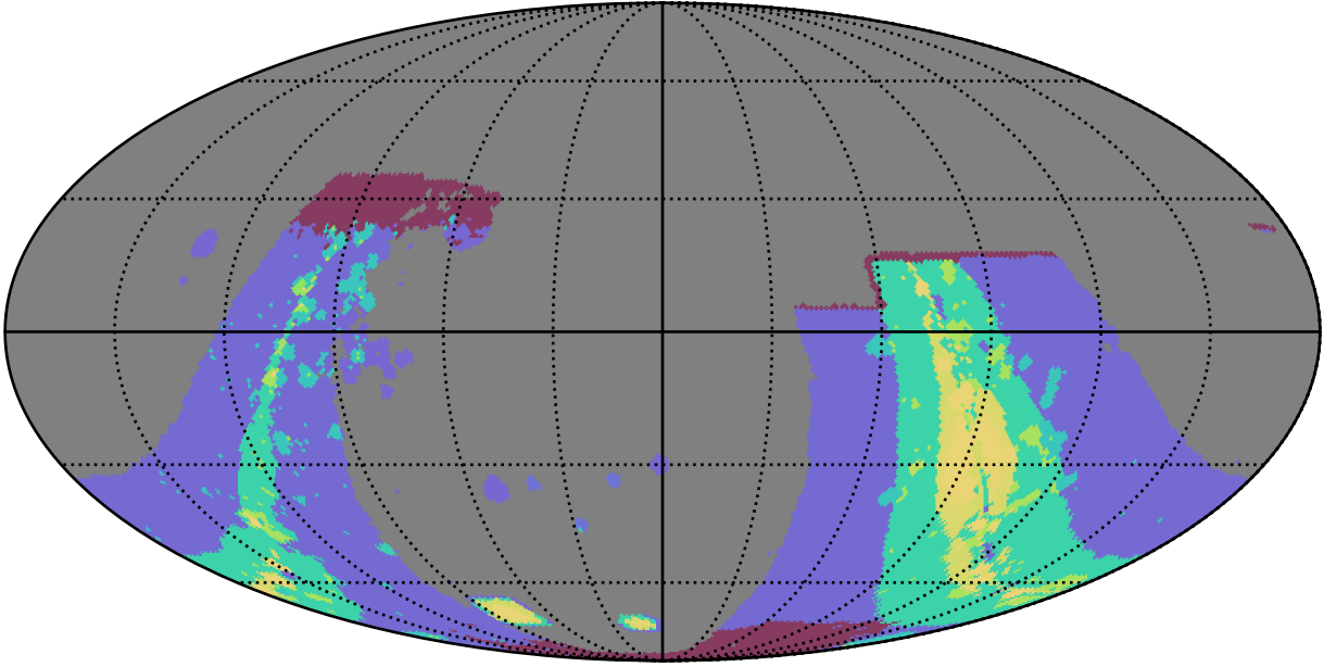
early_u_fpextra3.0_v3.4_10yrs : GalplaneFootprintMetric_combined_map_Tau_46_5
