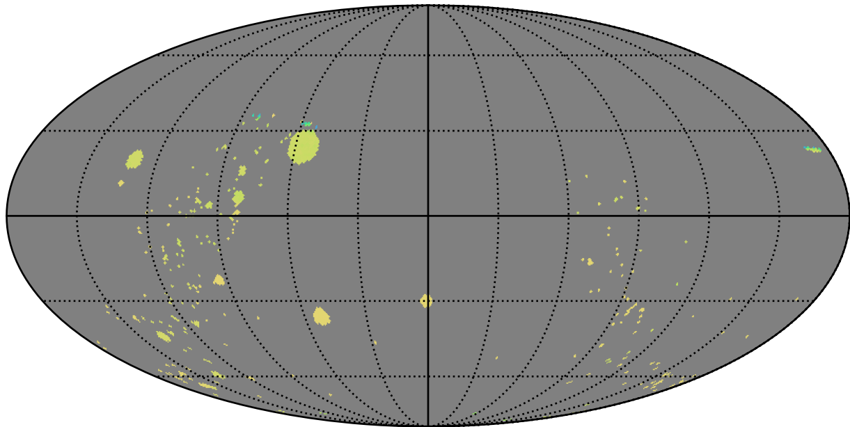
early_u_fpextra3.0_v3.4_10yrs : GalPlaneVisitIntervalsTimescales_open_clusters_map_Tau_46_5
