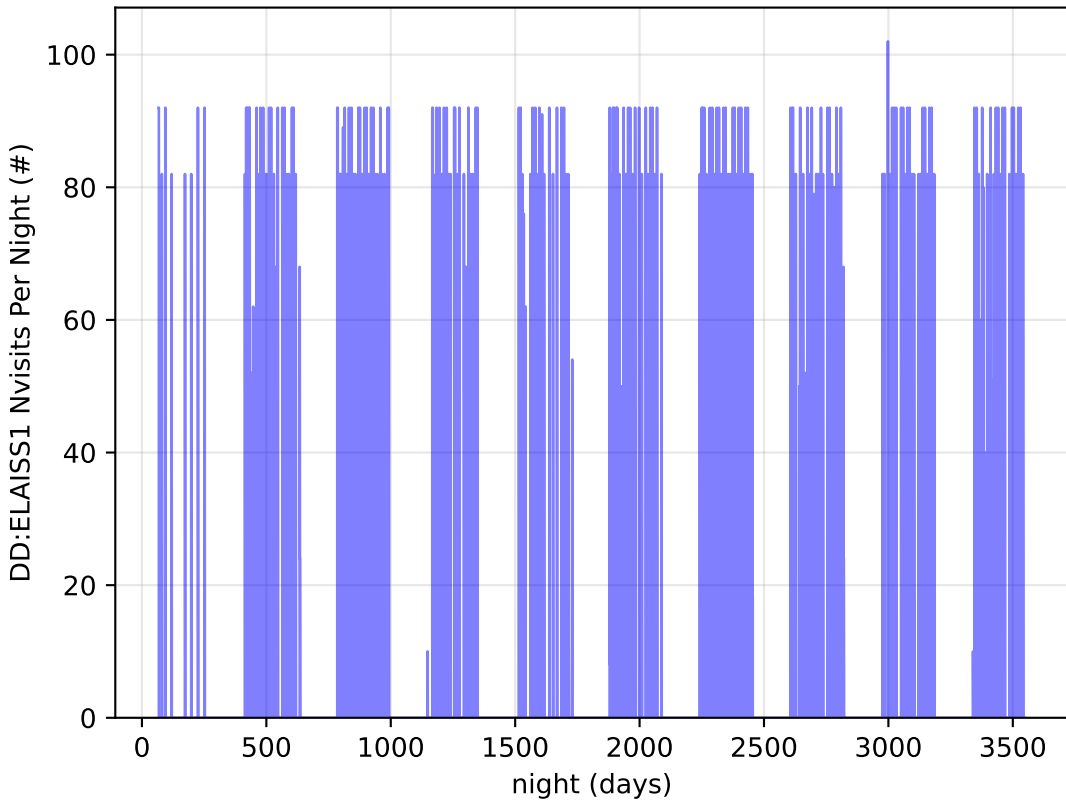
early_u_fpextra3.0_v3.4_10yrs all bands: DD:ELAISS1 Nvisits Per Night
