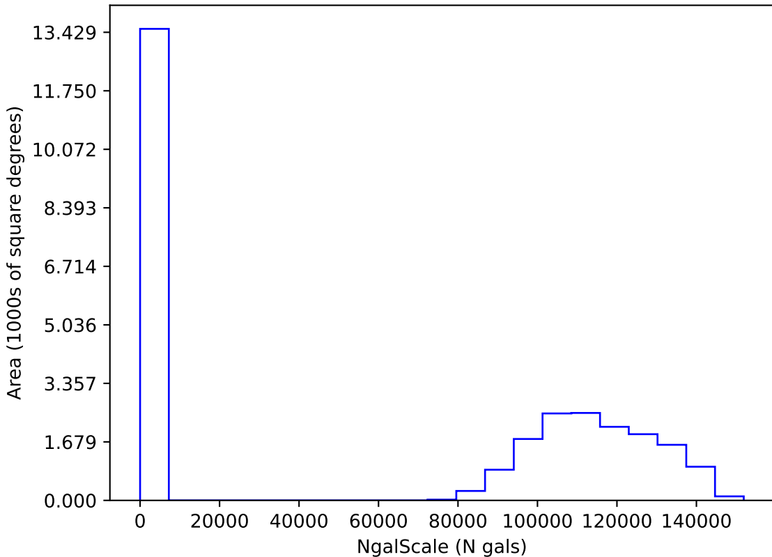
early_u_fpextra2.0_v3.4_10yrs i: NgalScale
