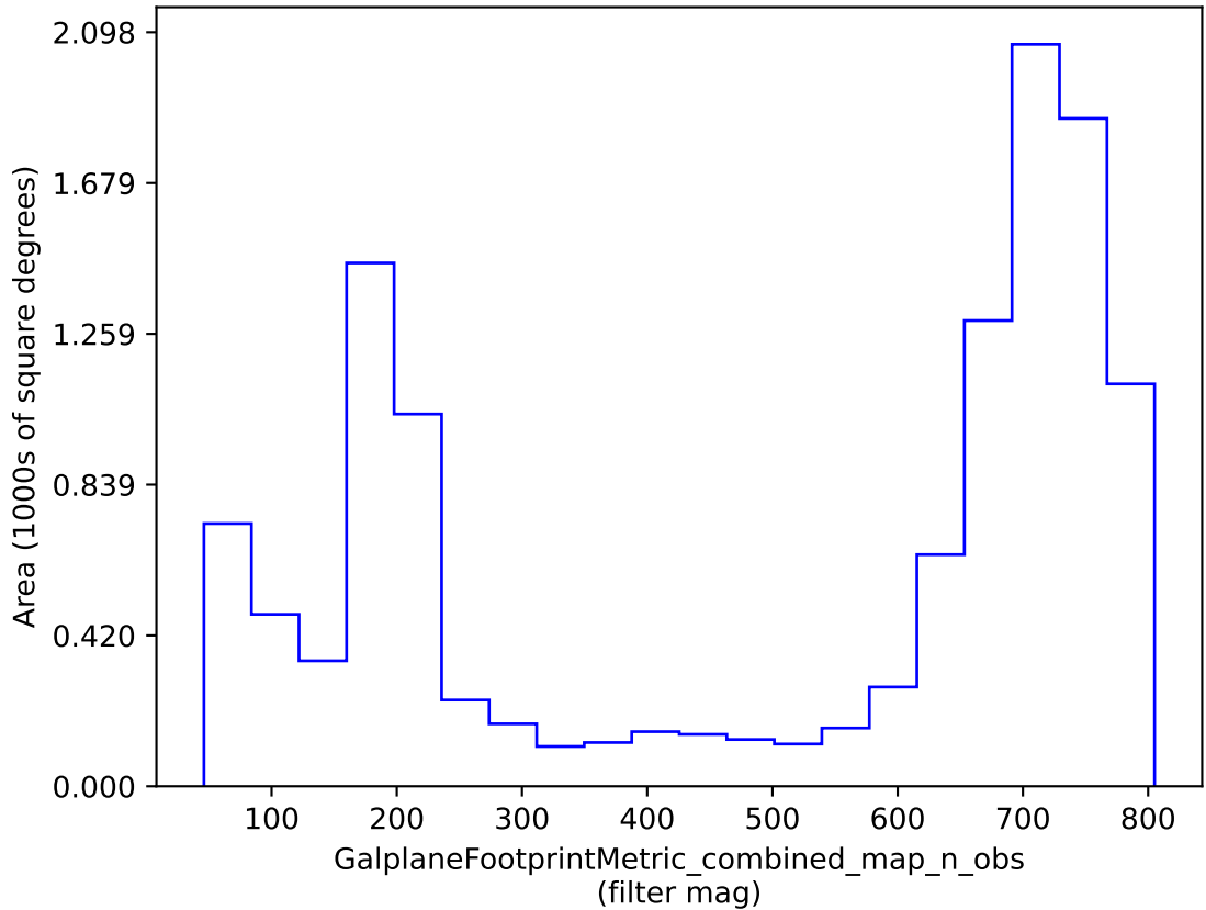
early_u_fpextra2.0_v3.4_10yrs : GalplaneFootprintMetric_combined_map_n_obs
