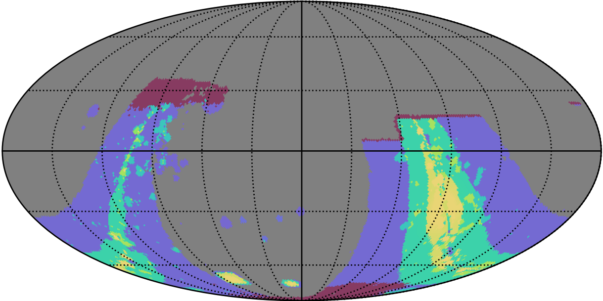
early_u_fpextra2.0_v3.4_10yrs : GalplaneFootprintMetric_combined_map_Tau_46_5
