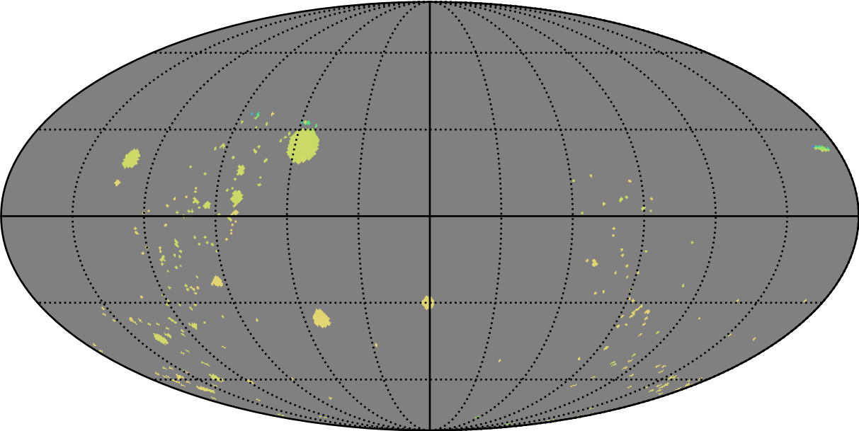
early_u_fpextra2.0_v3.4_10yrs : GalPlaneVisitIntervalsTimescales_open_clusters_map_Tau_46_5
