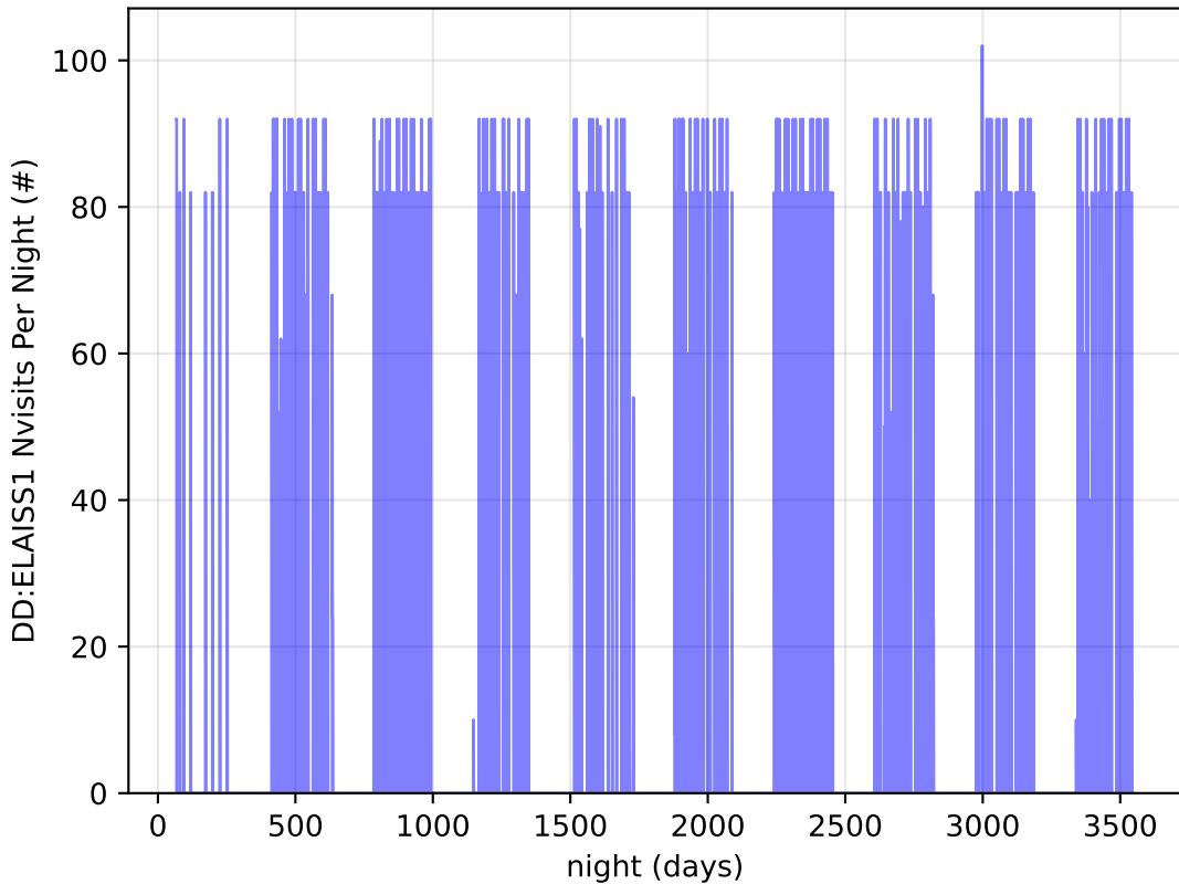
early_u_fpextra2.0_v3.4_10yrs all bands: DD:ELAISS1 Nvisits Per Night
