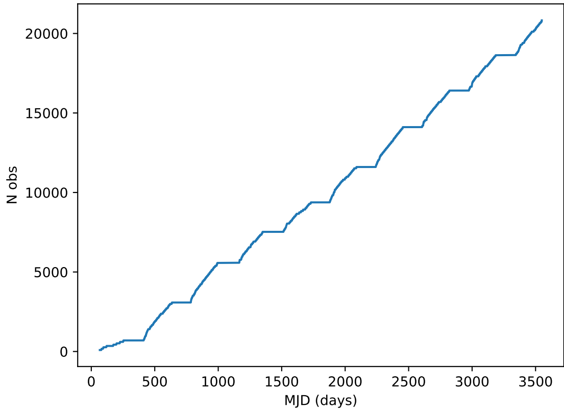
early_ss_template_fpextra5.0_v3.4_10yrs all bands: DD:ELAISS1 Cumulative NVisits
