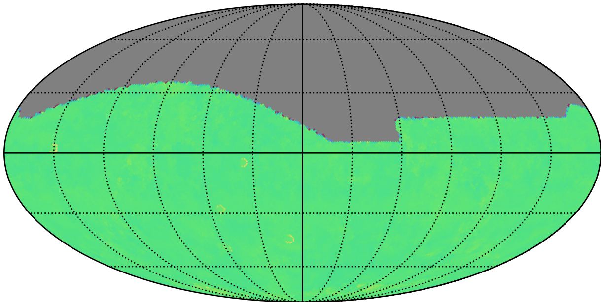
early_ss_template_fpextra3.0_v3.4_10yrs i: Kuiper rotTelPos
