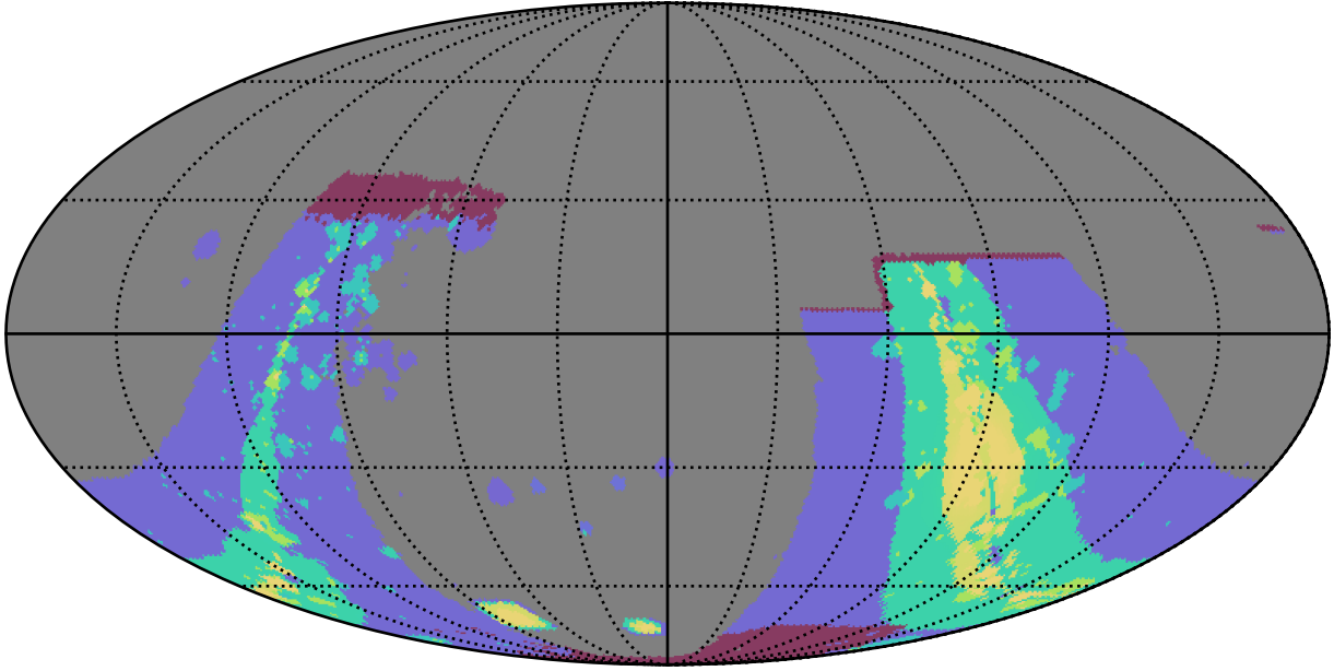
early_ss_template_fpextra3.0_v3.4_10yrs : GalplaneFootprintMetric_combined_map_Tau_46_5
