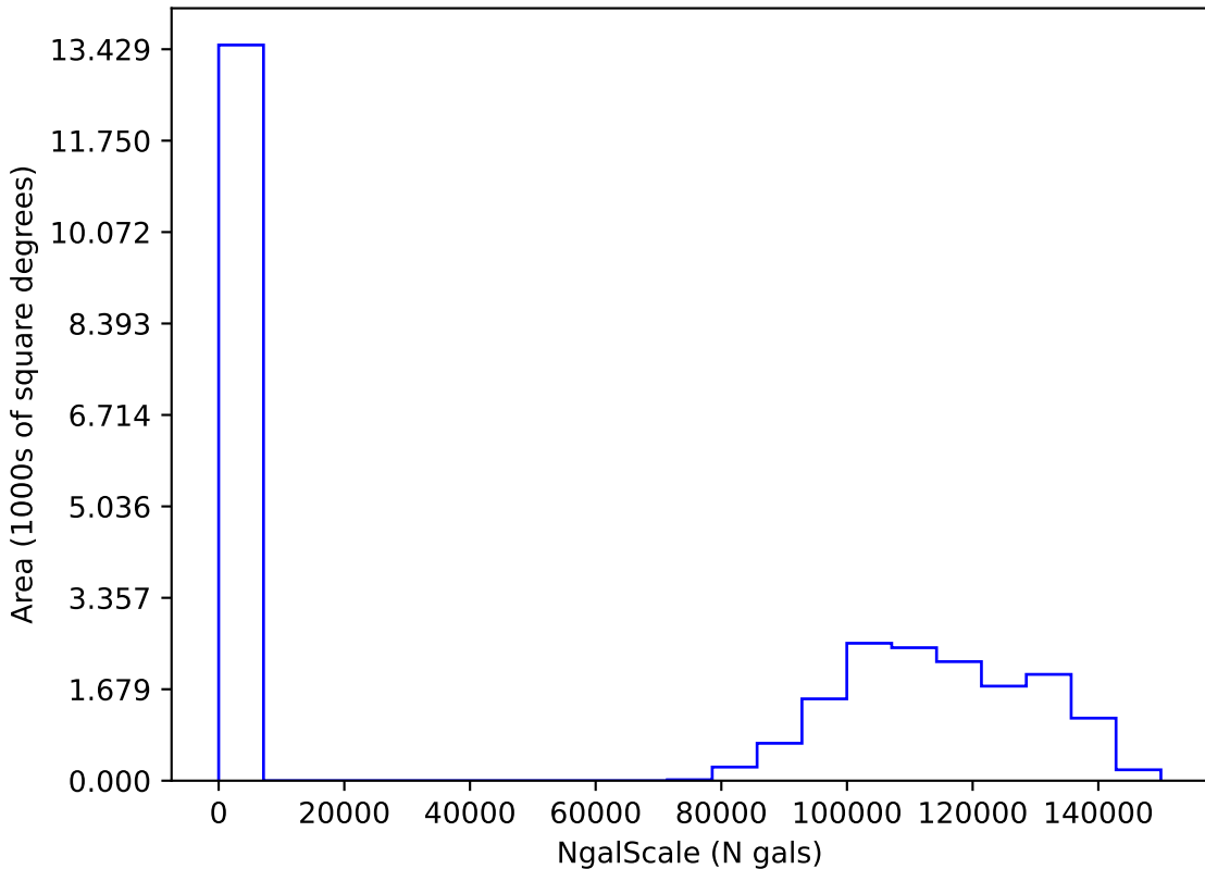
early_ss_template_fpextra1.5_v3.4_10yrs i: NgalScale
