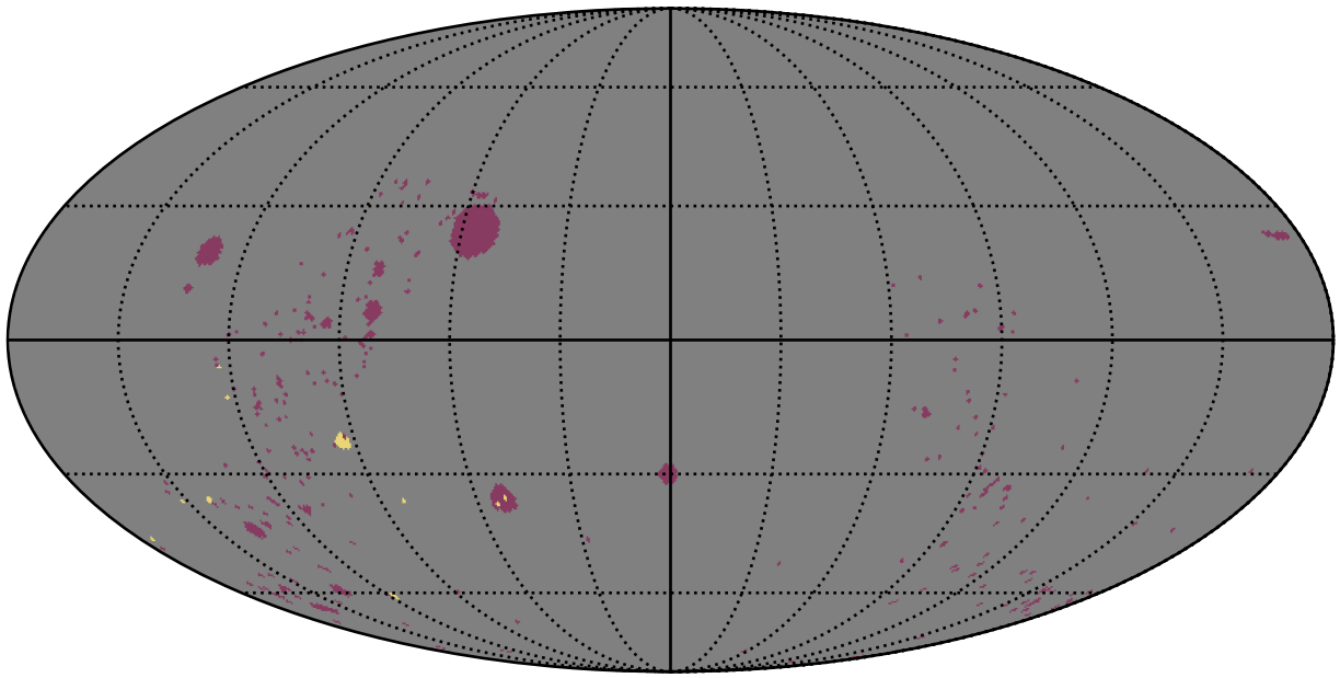
early_ss_template_fpextra1.5_v3.4_10yrs : GalplaneFootprintMetric_open_clusters_map_Tau_5_0
