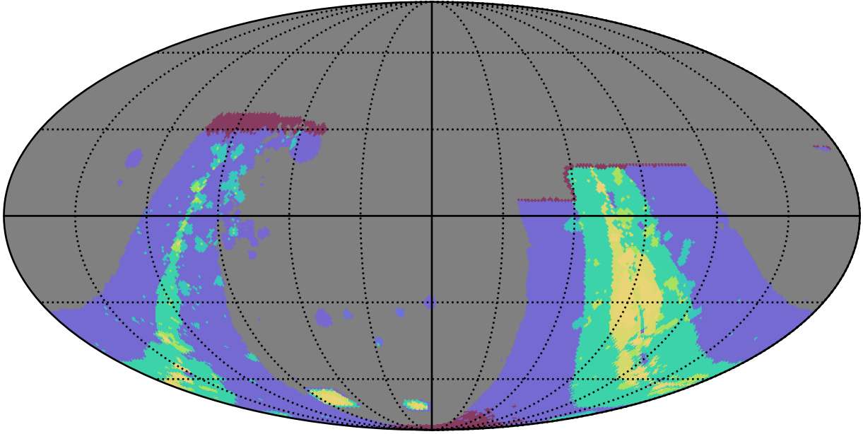
early_ss_template_fpextra1.5_v3.4_10yrs : GalplaneFootprintMetric_combined_map_Tau_73_0
