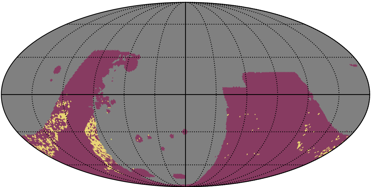
early_ss_template_fpextra1.5_v3.4_10yrs : GalplaneFootprintMetric_combined_map_Tau_5_0
