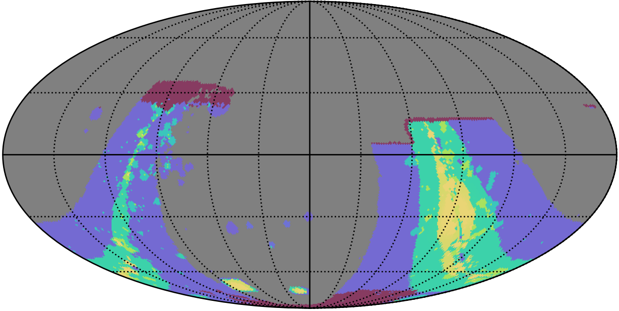
early_ss_template_fpextra1.5_v3.4_10yrs : GalplaneFootprintMetric_combined_map_Tau_46_5
