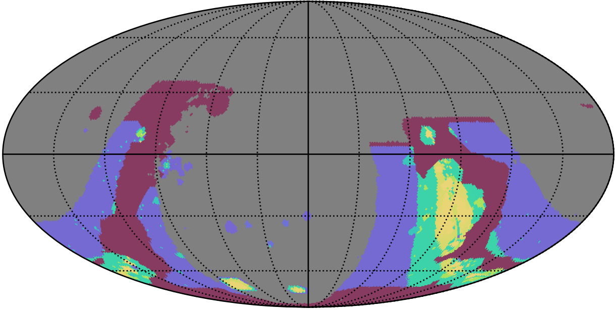
early_ss_template_fpextra1.5_v3.4_10yrs : GalplaneFootprintMetric_combined_map_Tau_11_0
