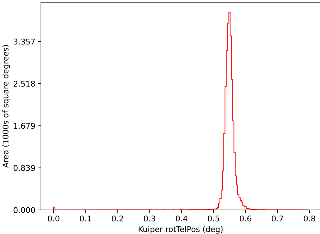
ddf_loaded_half_fl8_v3.4_10yrs i: Kuiper rotTelPos
