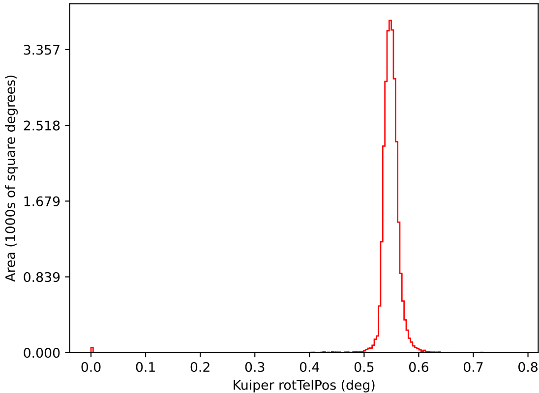
ddf_loaded_half_f14_v3.4_10yrs i: Kuiper rotTelPos
