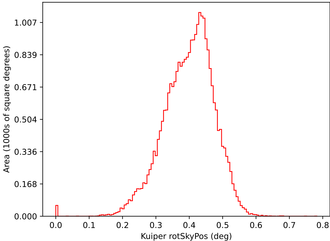
ddf_loaded_half_f14_v3.4_10yrs i: Kuiper rotSkyPos
