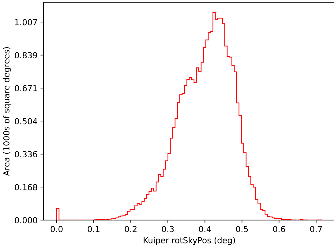
ddf_loaded_half_f12_v3.4_10yrs i: Kuiper rotSkyPos
