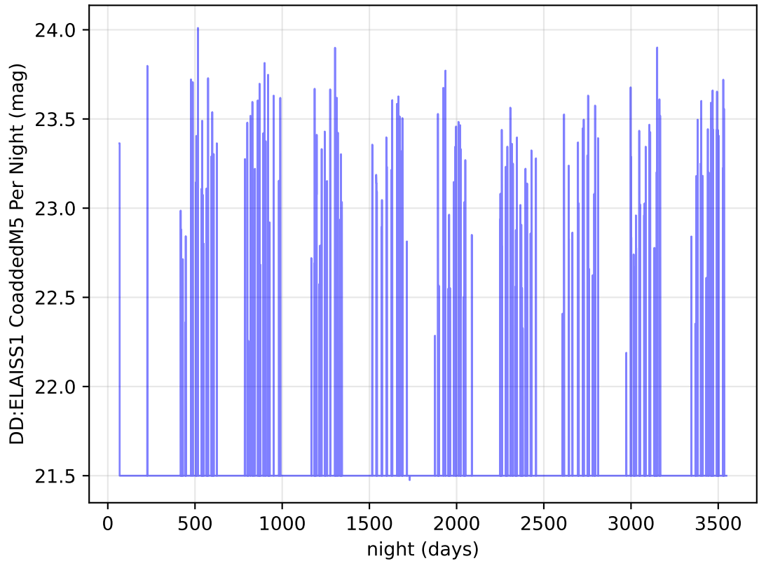
ddf_loaded_half_fl2_v3.4_10yrs y band: DD:ELAISS1 CoaddedM5 Per Night
