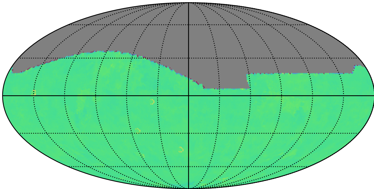
ddf_loaded_half_fl15_v3.3_10yrs i: Kuiper rotTelPos
