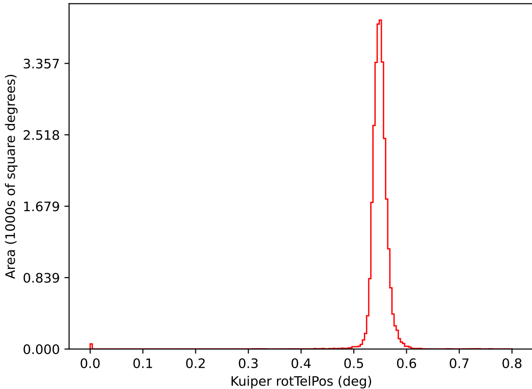
ddf_loaded_half_fl15_v3.3_10yrs i: Kuiper rotTelPos
