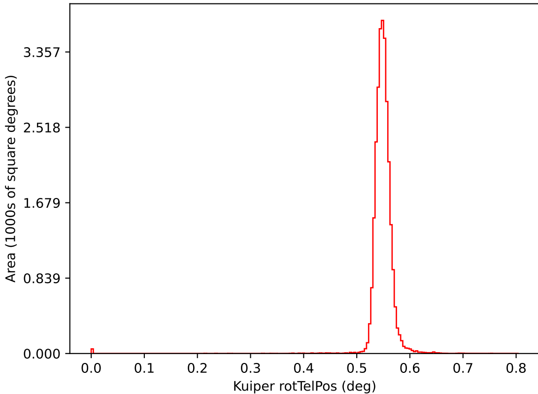
ddf_loaded_fl8_v3.4_10yrs i: Kuiper rotTelPos
