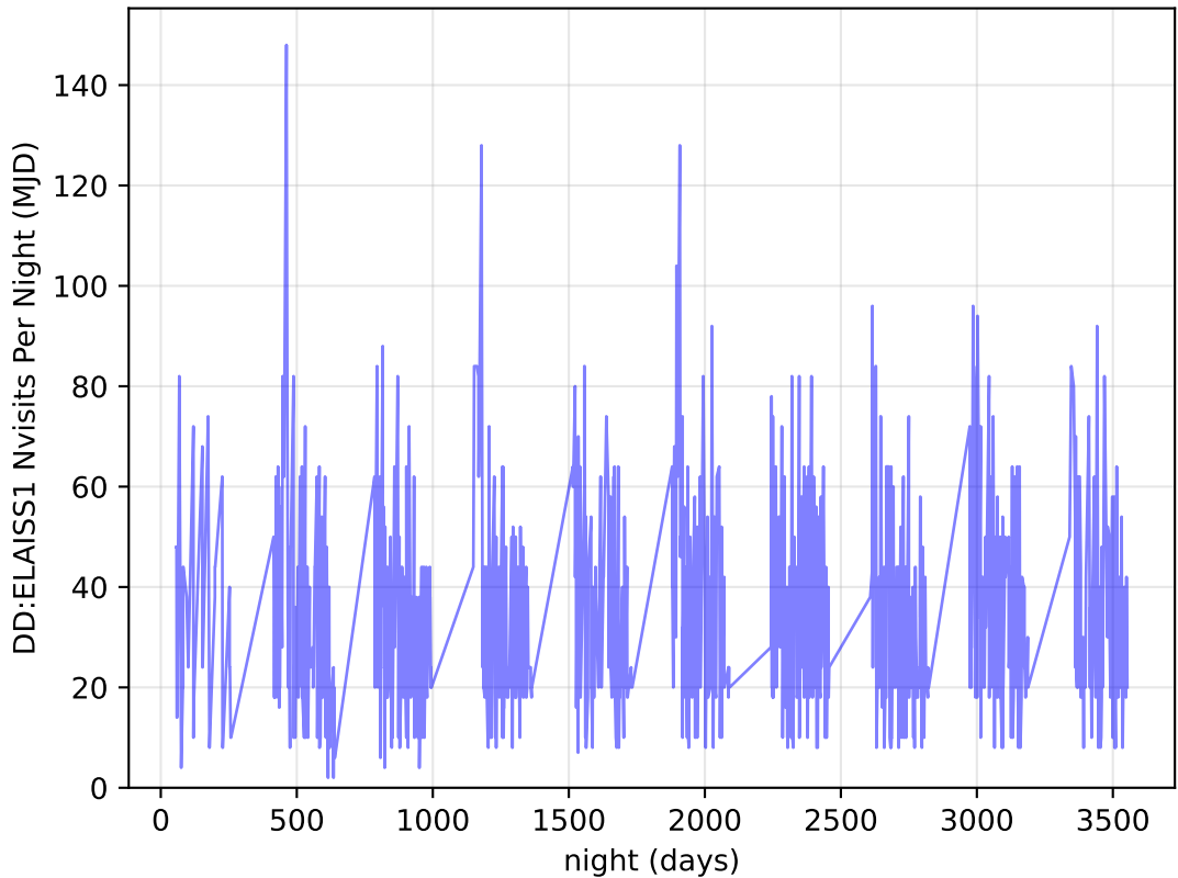
ddf_loaded_fl8_v3.4_10yrs all bands: DD:ELAISS1 Nvisits Per Night
