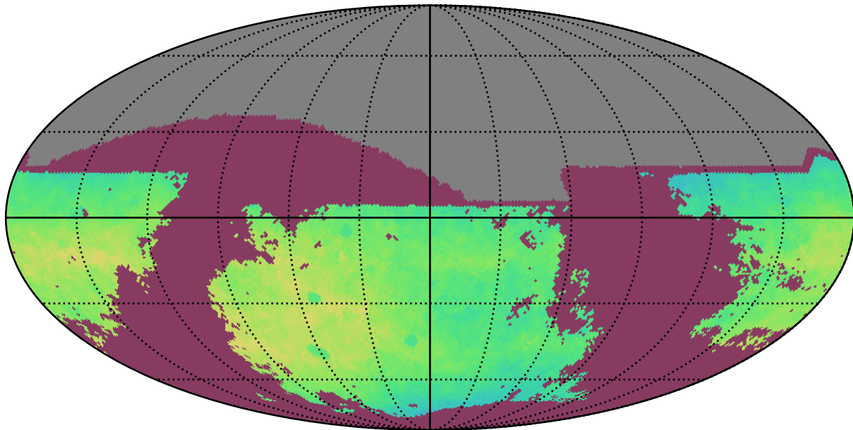
ddf_loaded_fl4_v3.4_10yrs i: NgalScale
