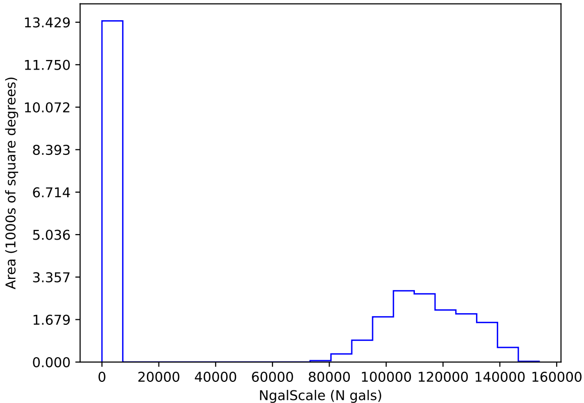
ddf_loaded_fl2_v3.4_10yrs i: NgalScale
