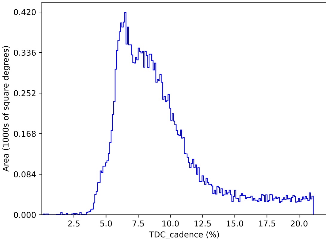
ddf_loaded_fl1_v3.4_10yrs : TDC_cadence
