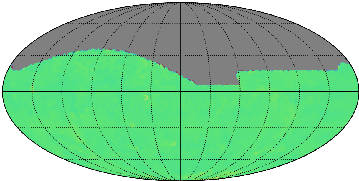
ddf_loaded_fl1_v3.4_10yrs i: Kuiper rotTelPos
