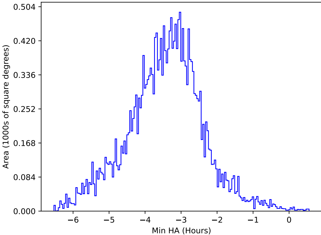
ddf_loaded_fl1_v3.4_10yrs All sky y band: Min HA
