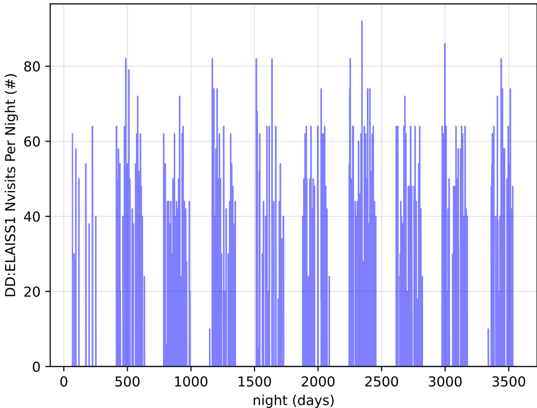
ddf_loaded_fl1_v3.4_10yrs all bands: DD:ELAISS1 Nvisits Per Night
