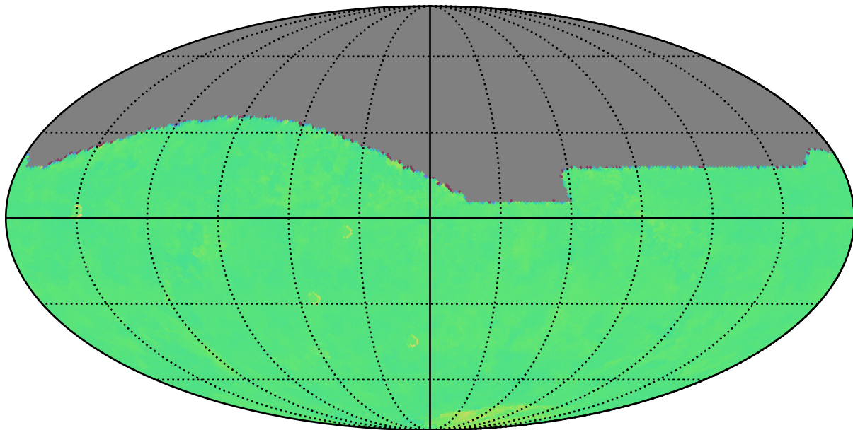
ddf_loaded_fl1_v3.3_10yrs r: Kuiper rotTelPos
