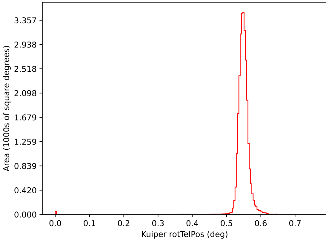
ddf_loaded_fl1_v3.3_10yrs i: Kuiper rotTelPos
