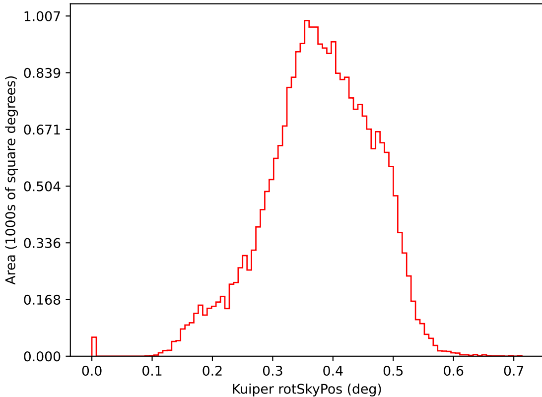
ddf_loaded_fl1_v3.3_10yrs i: Kuiper rotSkyPos
