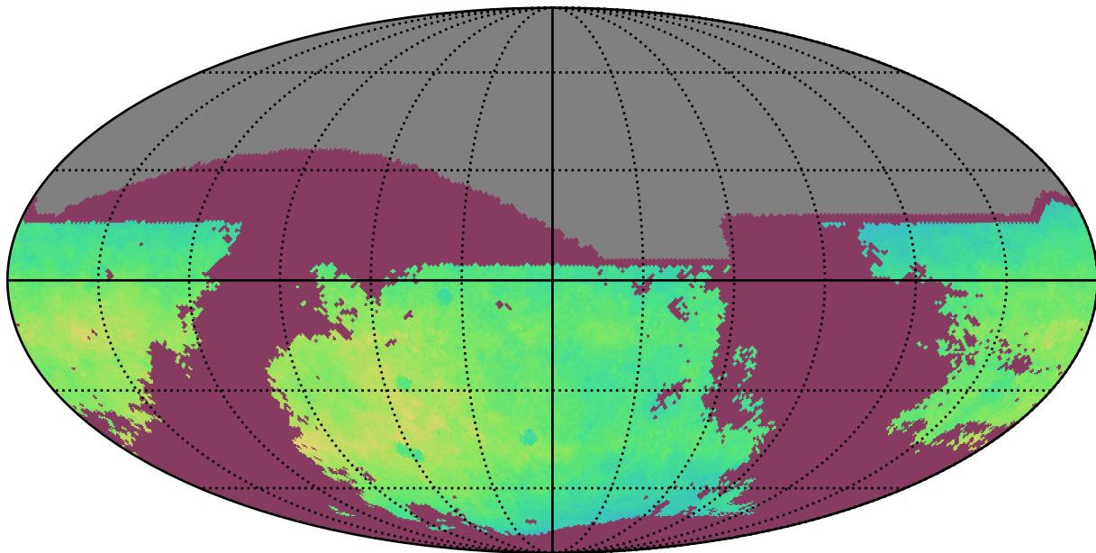
ddf_loaded_fl15_v3.4_10yrs i: NgalScale
