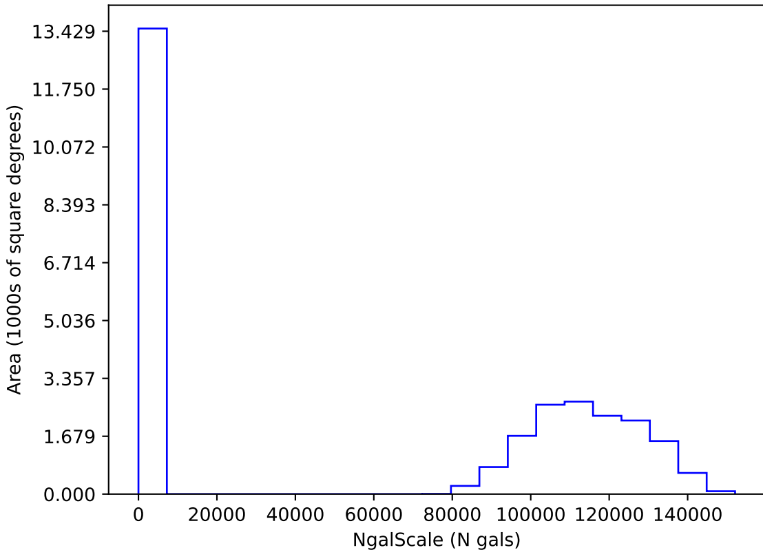
ddf_loaded_fl15_v3.4_10yrs i: NgalScale
