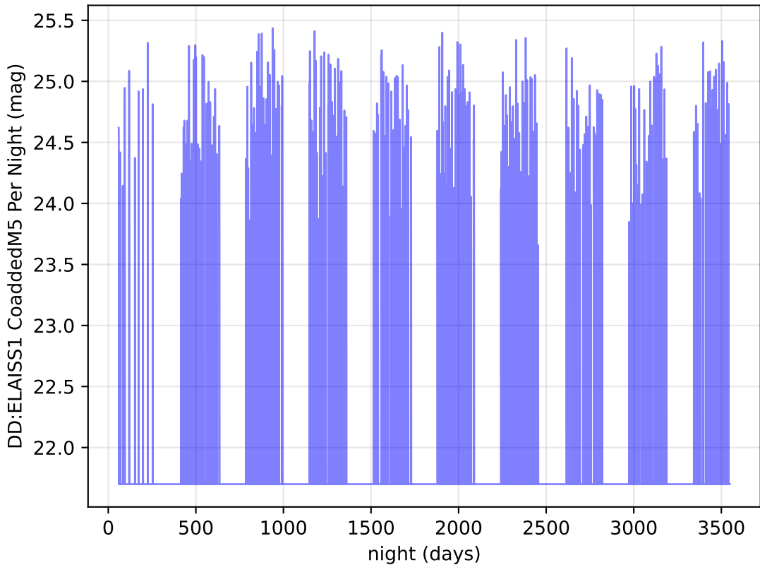
ddf_loaded_fl15_v3.4_10yrs z band: DD:ELAISS1 CoaddedM5 Per Night
