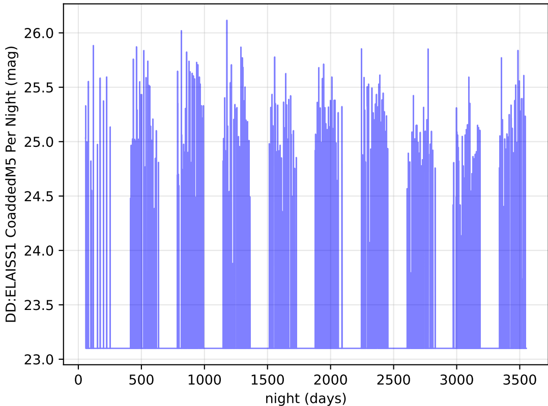
ddf_loaded_fl15_v3.4_10yrs i band: DD:ELAISS1 CoaddedM5 Per Night
