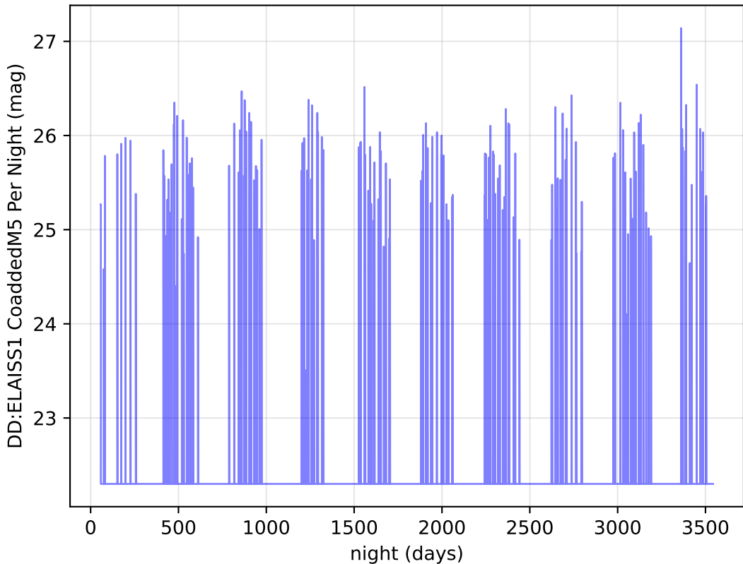
ddf_loaded_fl15_v3.4_10yrs g band: DD:ELAISS1 CoaddedM5 Per Night
