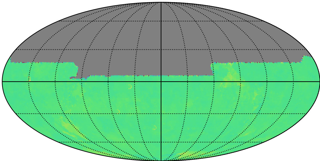
ddf_half_v3.4_10yrs y: Kuiper rotTelPos
