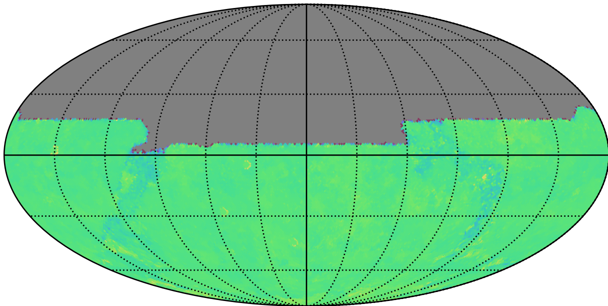
ddf_half_v3.4_10yrs u: Kuiper rotTelPos
